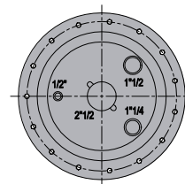
PARTICOLARE PASSO D'UOMO
